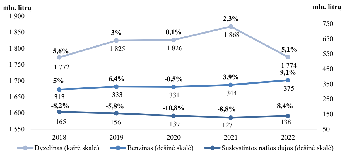
12 grafikas. Degalų pardavimų dinamika 2018–2022 metais*, mln. litrų ir proc.
