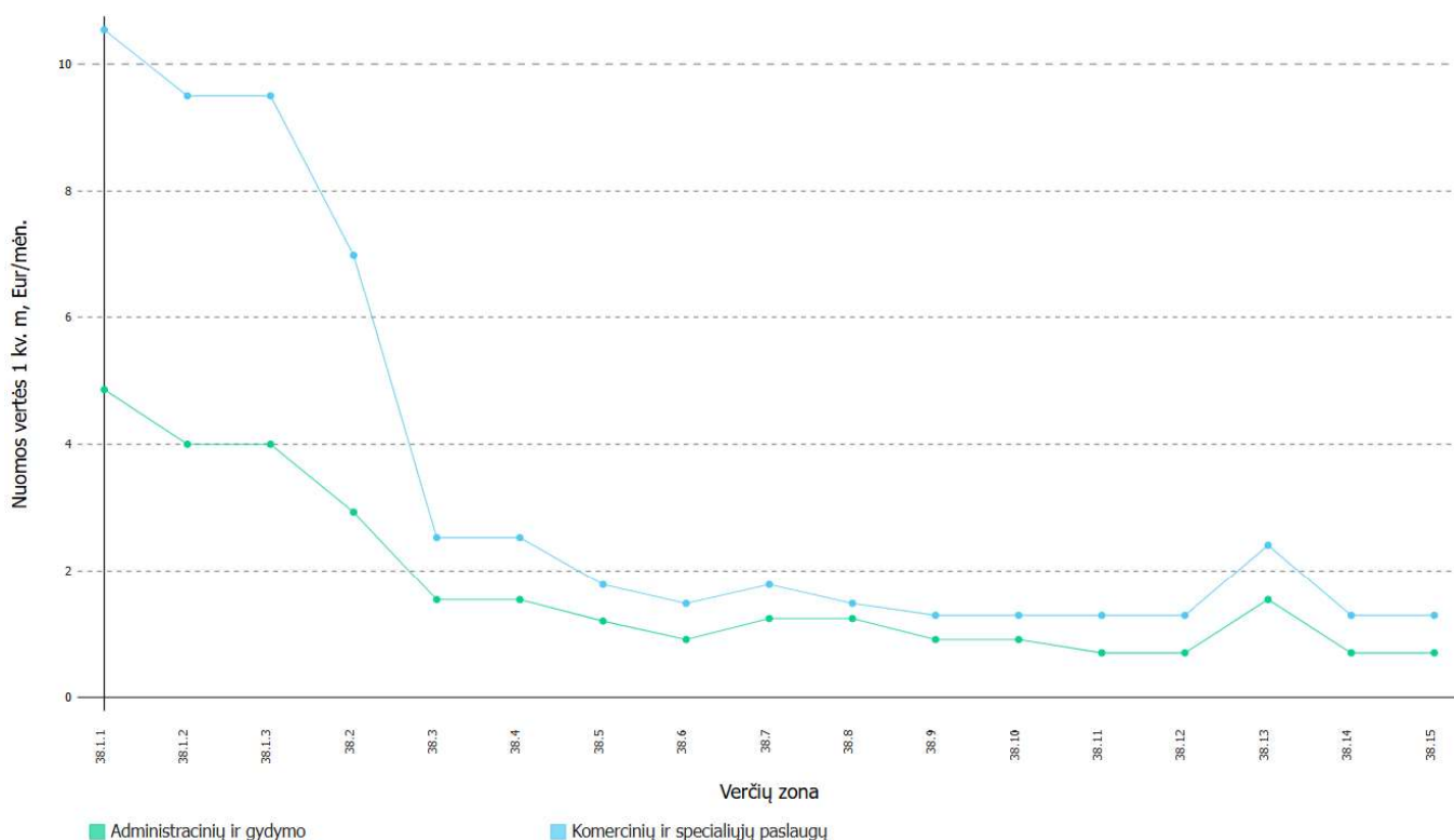
5.1 pav. Raseinių rajono savivaldybės nekilnojamojo turto vidutinių nuomos verčių vertinimo modelių vertikali–horizontali patikra
