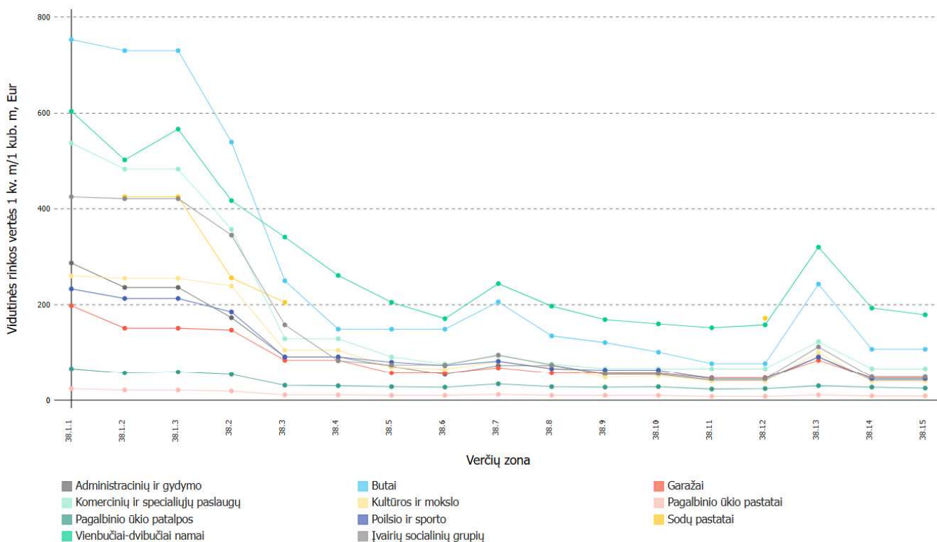
4.1 pav. Raseinių rajono savivaldybės nekilnojamojo turto vertinimo modelių vertikali–horizontali patikra
