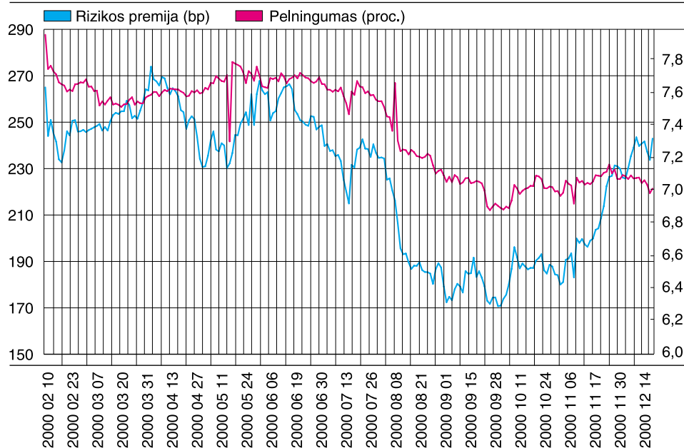
Lietuvos Respublikos Vyriausybės 7,75 proc. obligacijų, išperkamų 2005 metais pelningumas ir rizikos premija nuo jų platinimo pradžios 2 grafikas
